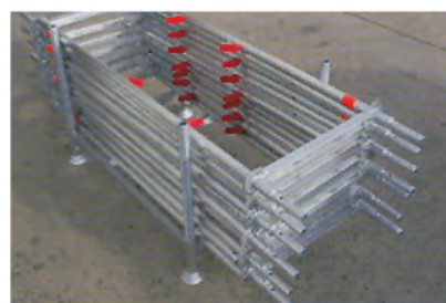
Almacenamiento y transporte usando el pallet 125
